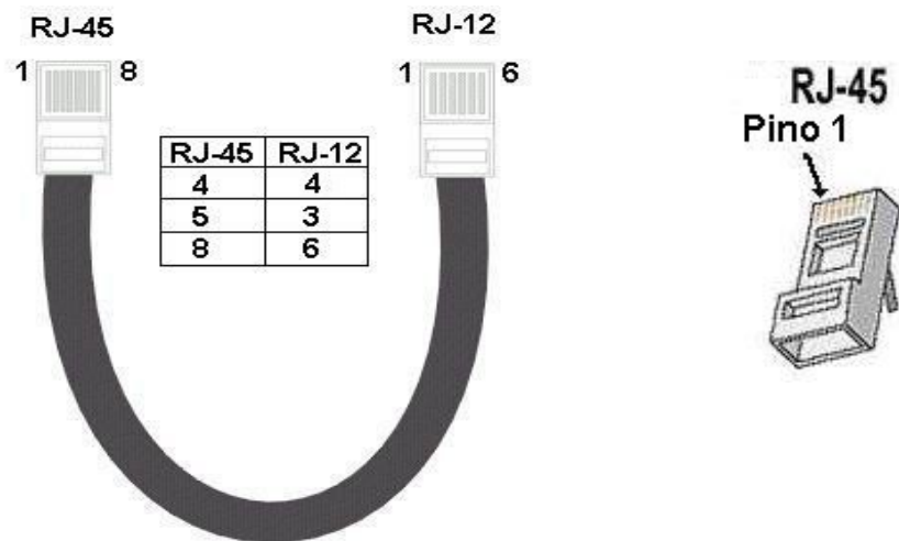
Pinagem do cabo URANET com microterminais utilizando conector RJ-45.
