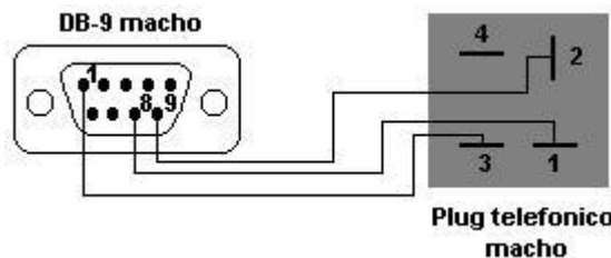
DB-9 macho
